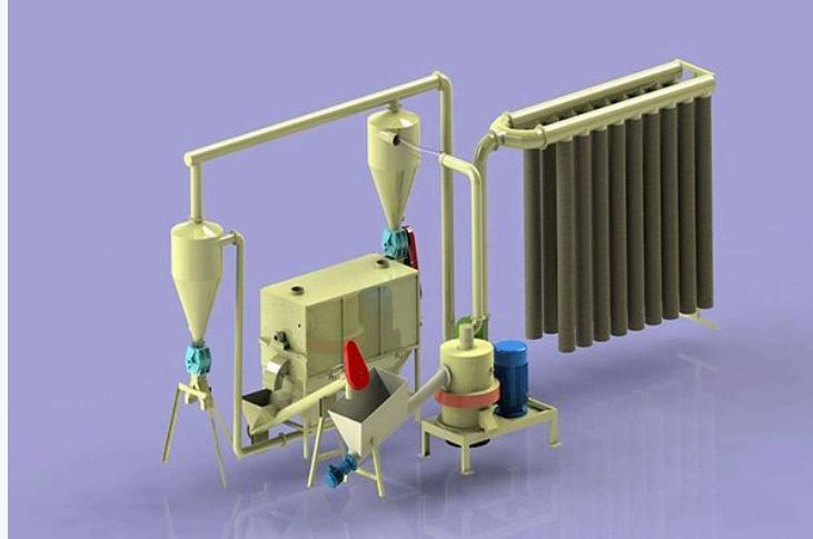
🌲 Máquina vertical de polvo de madera · Operación eficiente y estable
